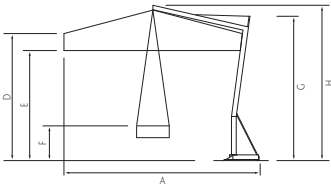
DUO met ALUMINIUM VOET
