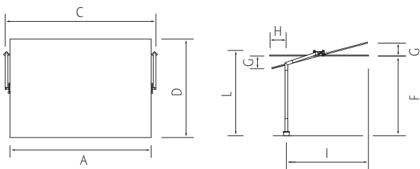
FLEXY MET OPZETSTUK OP BETONVERANKERING
