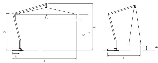
CAPRI met ALUMINIUM VOET
