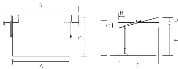
AFMETINGEN (CM) FLEXY
