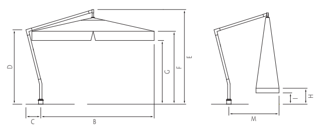
CAPRI met OPZETSTUK OP BETONVERANKERING
